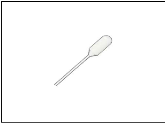
品名 スポイトエコノミー 0.5mL 材質:LDPE(低密度ポリエチレン) 長さ:65mm 滴下量:48 \mu L 小箱入数:2,000 大箱入数:20,000
